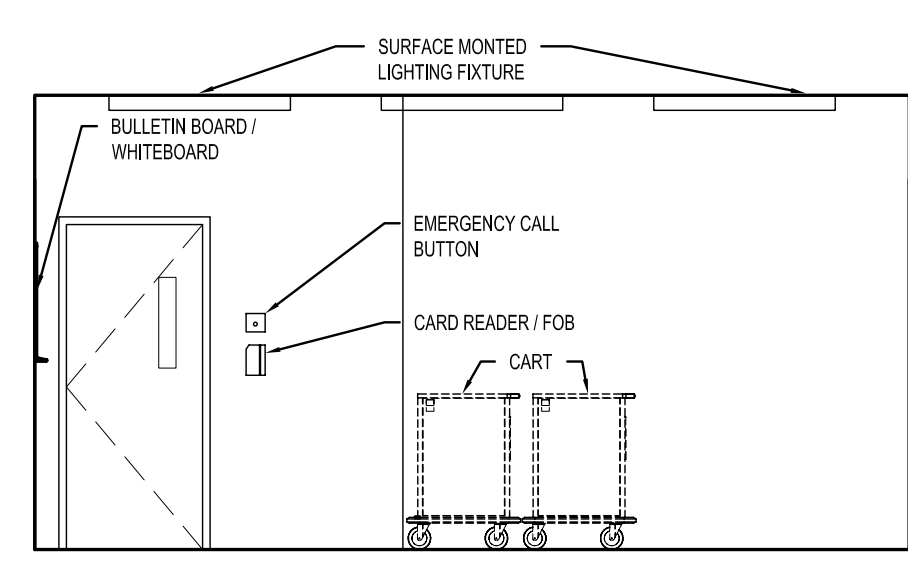
1E ELEVATION 1:50
