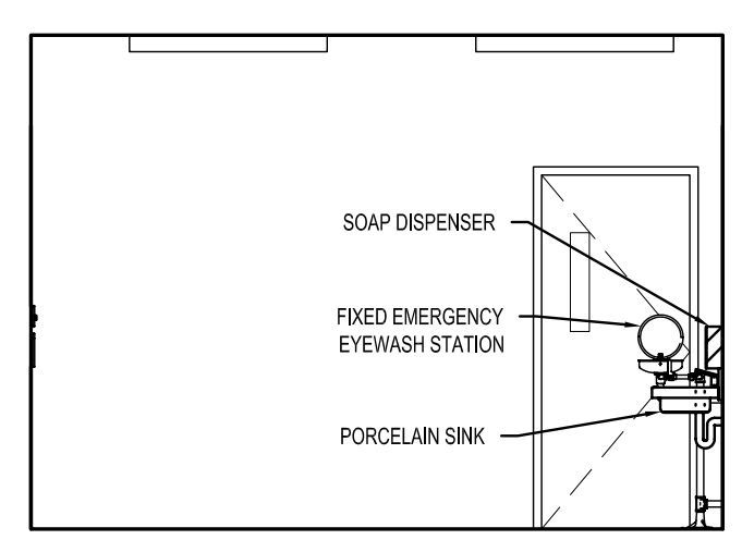
4D ELEVATION 1:50
