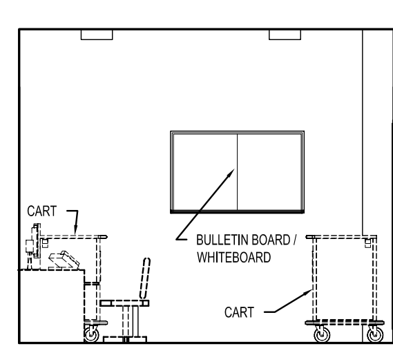
1B ELEVATION 1:50
