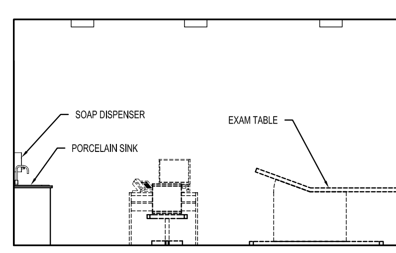
2B ELEVATION 1:50
