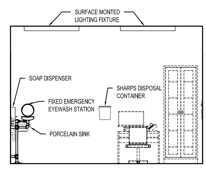
4E ELEVATION 1:50
