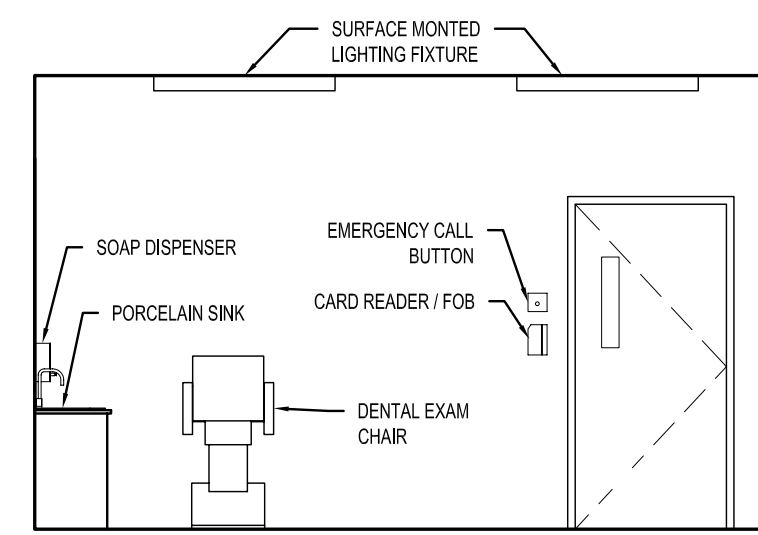
3E ELEVATION 1:50
