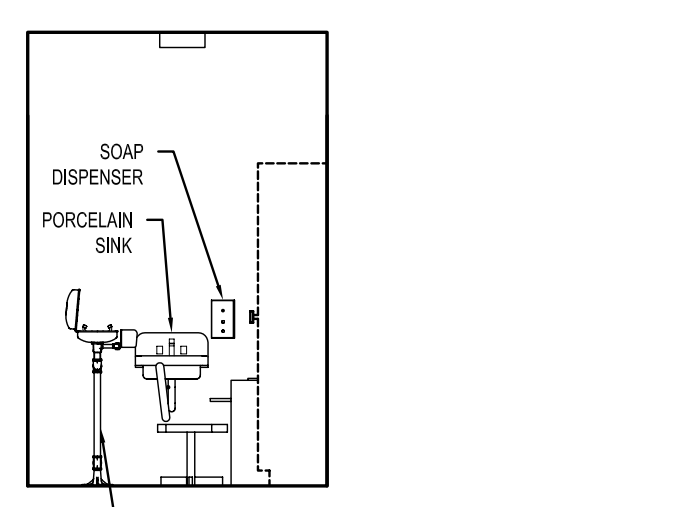
4B ELEVATION 1:50
