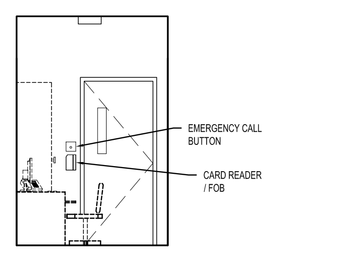
4C ELEVATION 1:50
