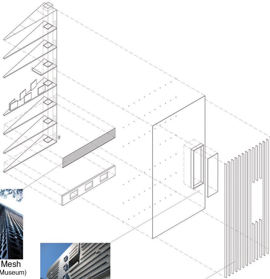
AXONOMETRIC
