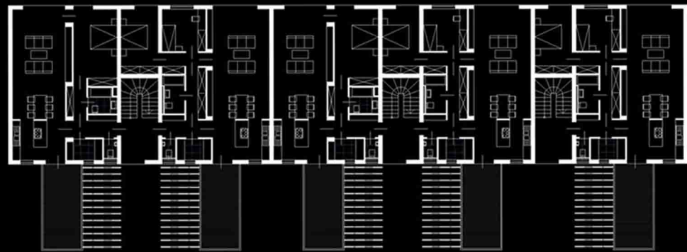
EMELETI ALAPRAJZ
