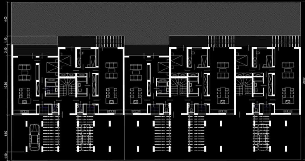
FÖLDSZINTI ALAPRAJZ
