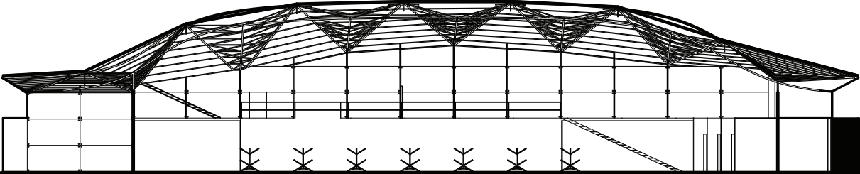
LONGITUDINAL SECTION
