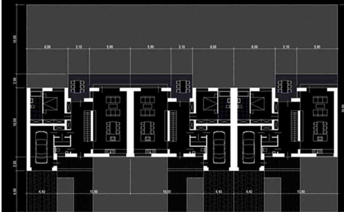
FÖLDSZINTI ALAPRAJZ
