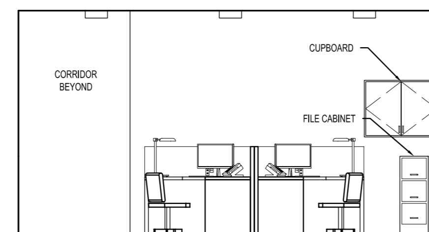
1B ELEVATION 1:50
