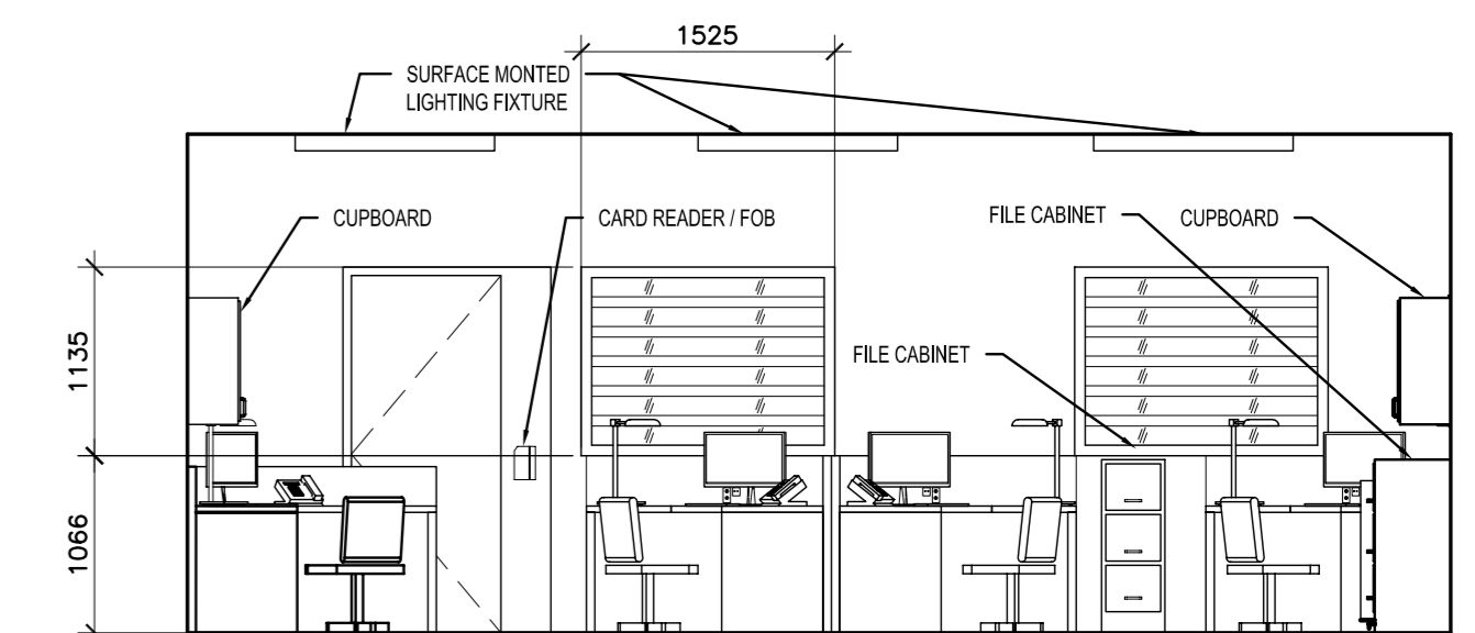
1E ELEVATION 1:50
