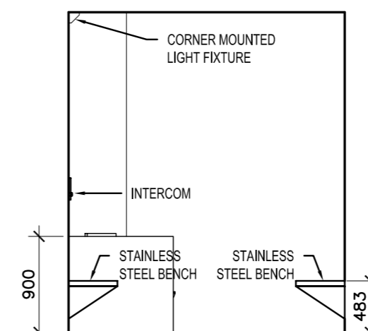
4B ELEVATION 1:50
