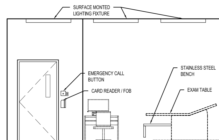
1E ELEVATION 1:50
