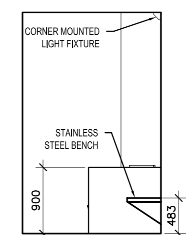
5B ELEVATION 1:50
