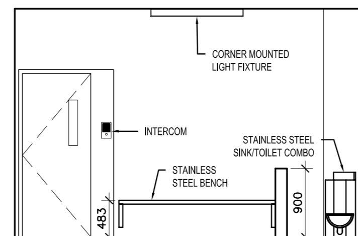
4D ELEVATION 1:50
