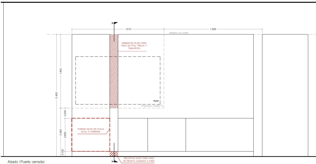
Alzado (Puerta cerrada)
