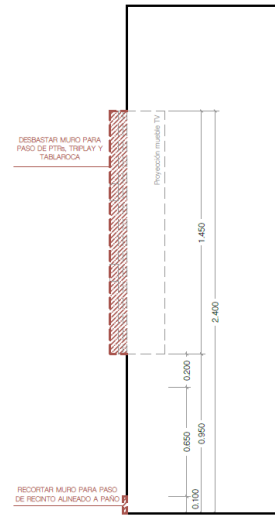
Corte AA (Por muro a desbastar)
