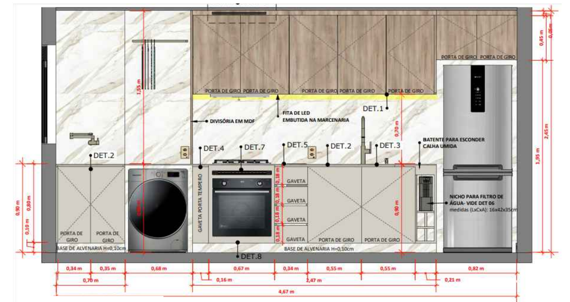
4 Elevação- Cozinha Esc 1/125
