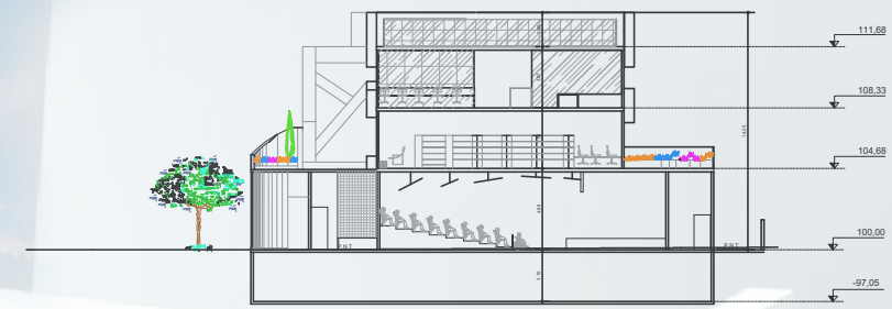
CORTE AA
