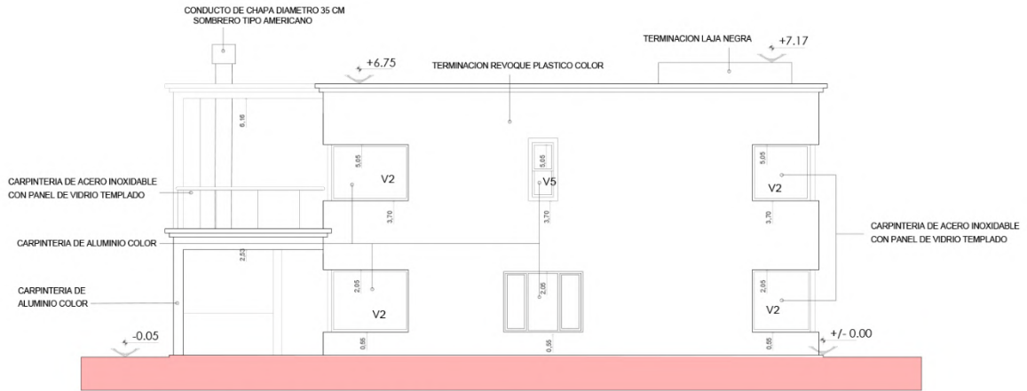
VISTA LATERAL IZQUIERDOESC. 1:100
