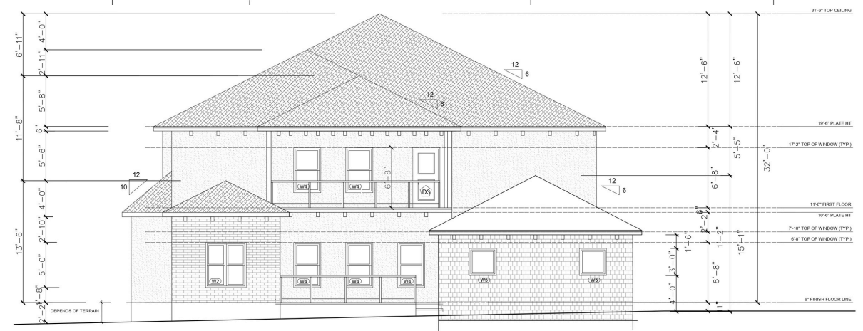
1 RIGHT ELEVATION
